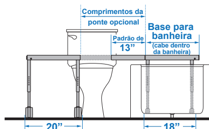
Diagrama da base de transferência
