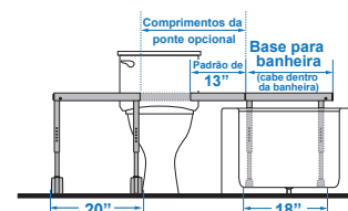
Diagrama da base de transferência
