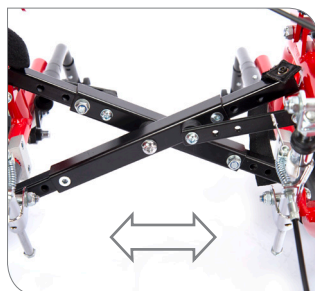
Estrutura em x com largura ajustável
