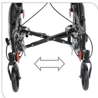
Estrutura em x com largura ajustável
